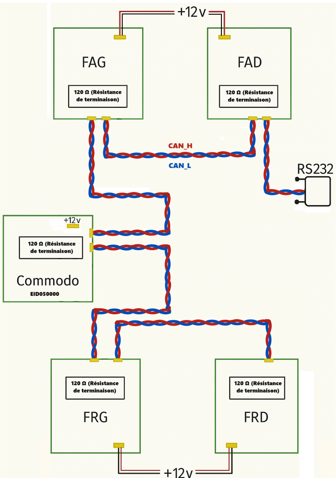
Figure -19- Architecture du réseau CAN du module CAN01A avec les résistances de terminaison et alimentation 12V.
