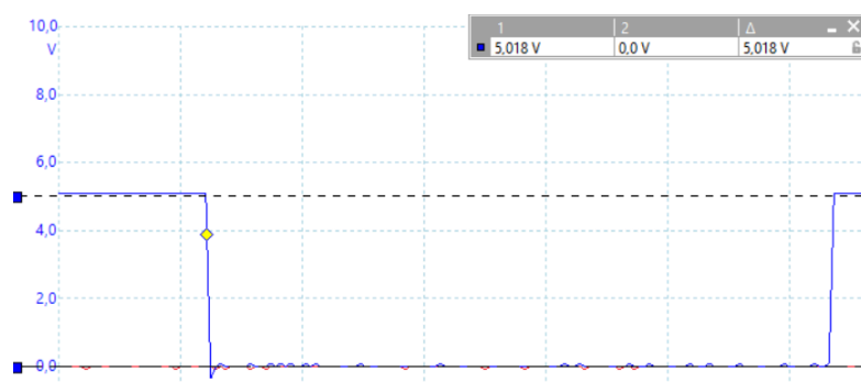
Figure -21- visualisation de signal d'interruption sur le picoscope.
